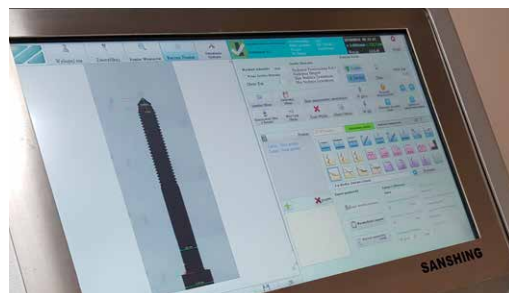
Pomiar twardości i kontrola wymiarów Hardness test and dimensional inspection
