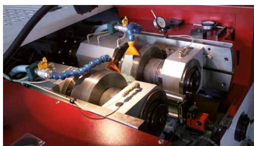
Walcowanie gwintów Thread rolling
